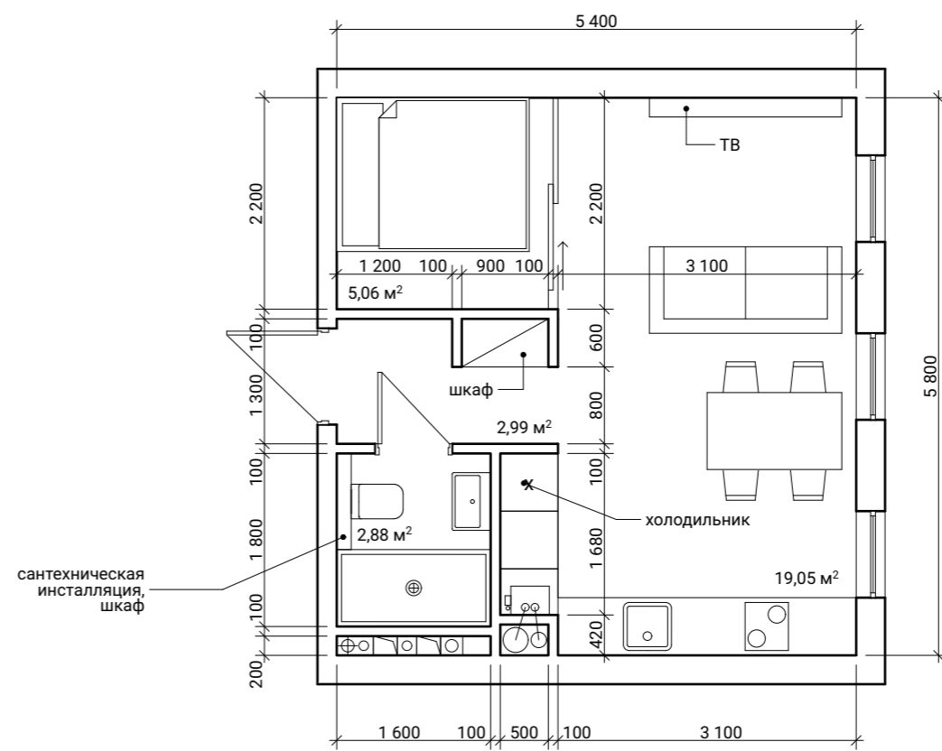
план расстановки мебели и оборудования
